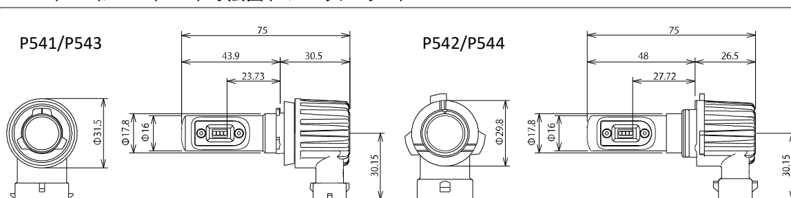
P541(P543)/P542(P544) 寸法図(コンパクトスター)
