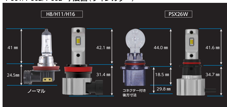
P561/P562/P552 寸法図(ツインカラー)
